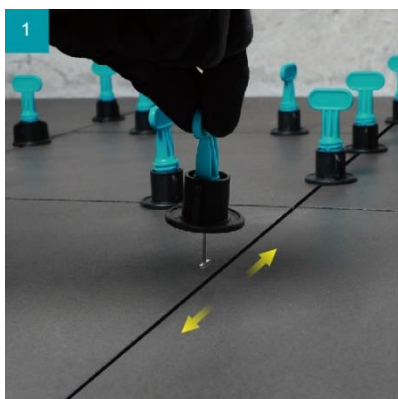
1. Sisestage T-spin ots paralleelselt plaadivuugi vahele
