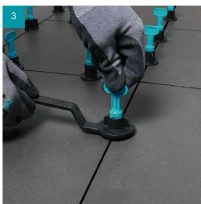
3. Pingutage alumist mutrit kuni tasapind on saavutatud
