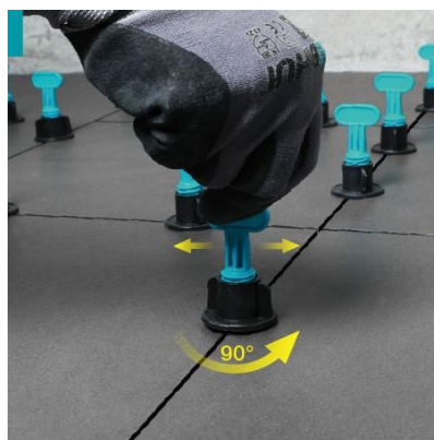
4. Hiljemalt 24h jooksul vabastage alumine koonus, keerake T-spin ots 90 kraadi tagasi ja eemaldage T-spin
