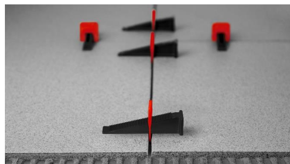
2. Paigalda kõrvale uus plaat ja sisesta kiil
