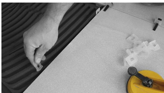
1. Paigalda plaatimisankur plaadi serva alla
