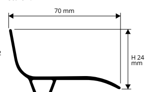
PETFXAA 70 scale 1:2
