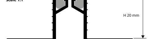
PFXAL/OT 20 scale 1:1
