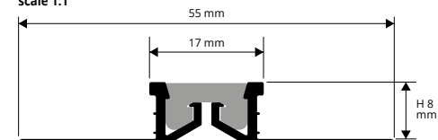
PFXAL/OT 08 scale 1:1
