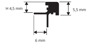
PKLQ... 045 scale 1:1
