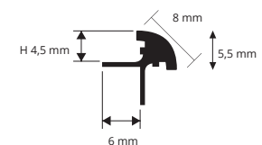
PKLJ... 045 scale 1:1
